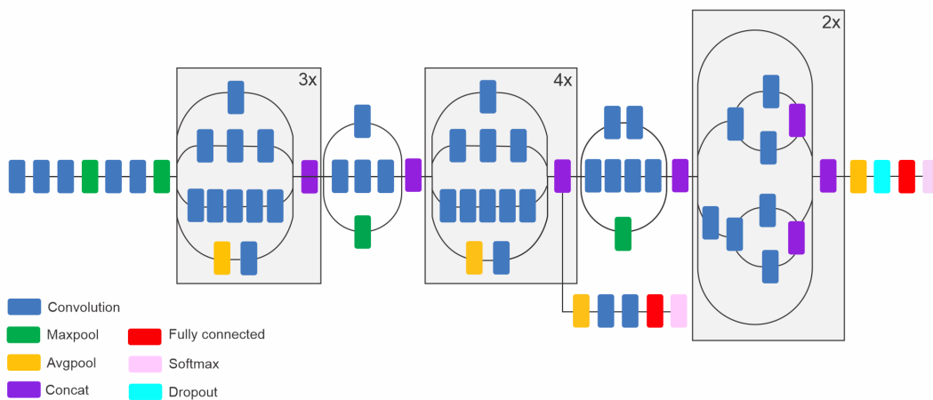
FIGURA 2.7: Versión simplificada de InceptionV3. [12]
