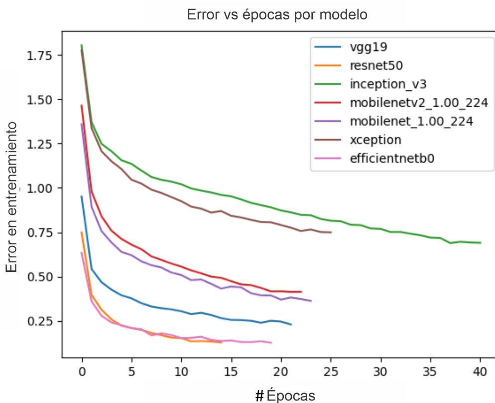
FIGURA 5.1: Gráfica comparativa de la pérdida entre todos los modelos a estudiar
