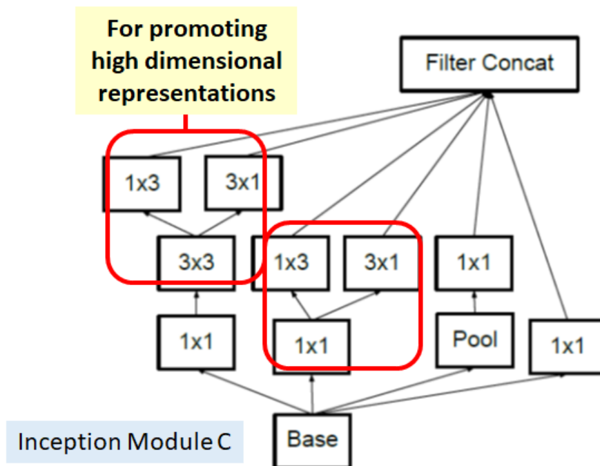
FIGURA 2.6: Reducción de la dimensionalidad del InceptionV3. [12]
