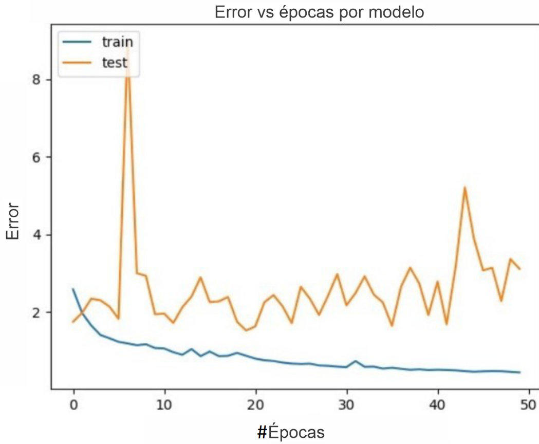
FIGURA 5.14: Gráfica comparativa de la pérdida de entrenamiento y testing
