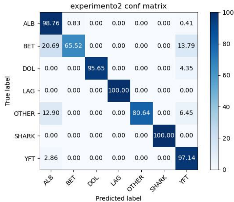
FIGURA 5.3: Matriz de confusión generada por el experimento #2 en porcentajes
