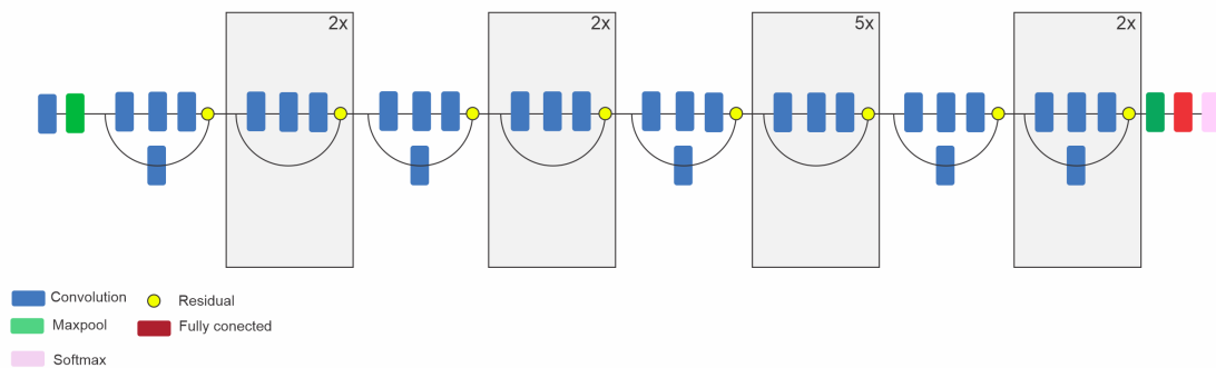
FIGURA 2.8: Versión simplificada de ResNet50. [12]
