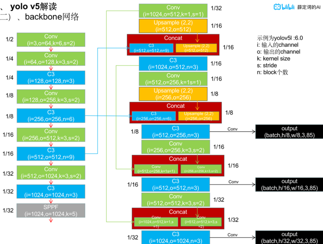
FIGURA 2.10: Representación de la arquitectura YOLOV5 [18]
