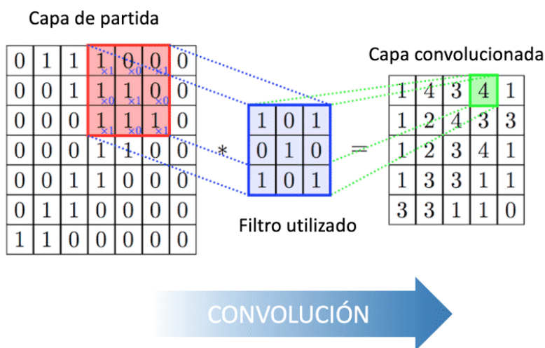
FIGURA 2.2: Proceso de convolución simplificado[8].
