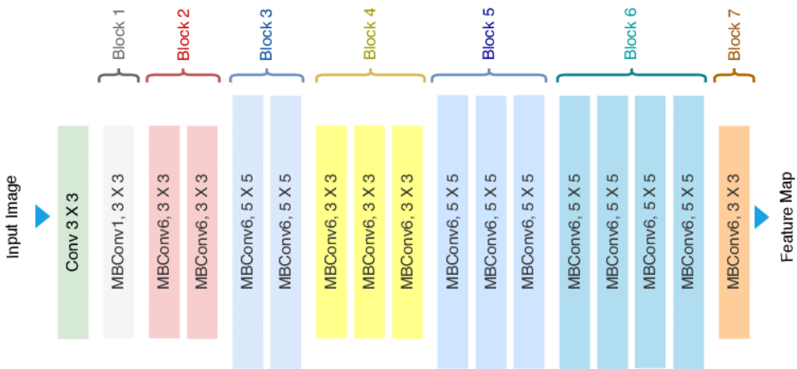
FIGURA 2.9: Versión simplificada de EfficientNetB0. [16]
