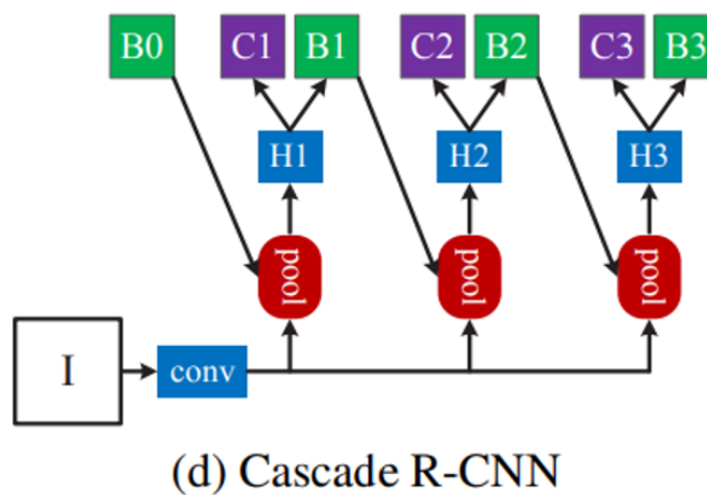
FIGURA 2.12: Representación de la arquitectura Cascade RCNN [20].
