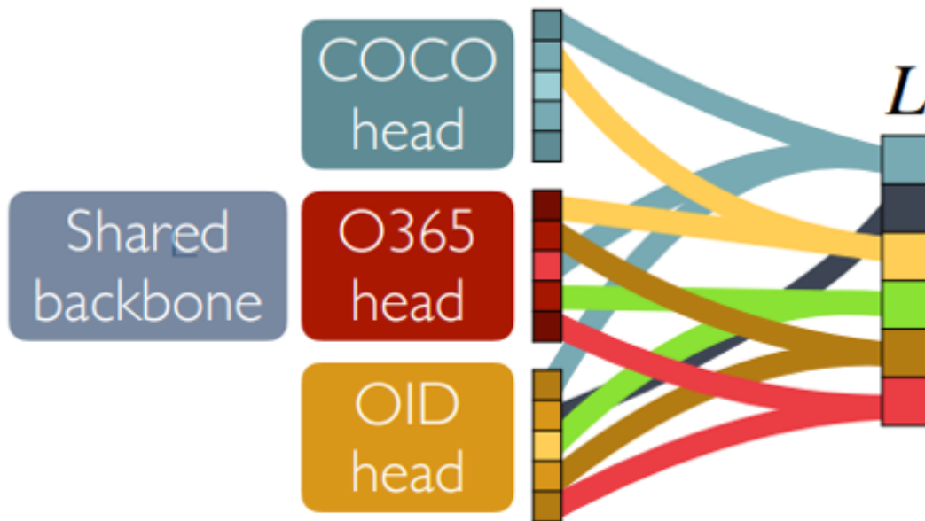
FIGURA 2.11: Representación de la arquitectura UniDet [19].
