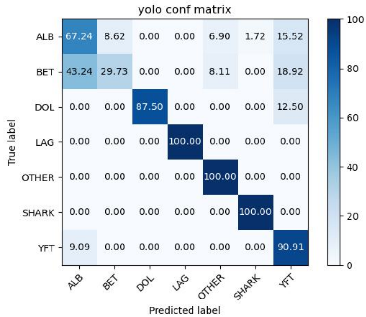
FIGURA 5.11: Matriz de confusión para pruebas del pipeline con Yolov5 preentrenado
