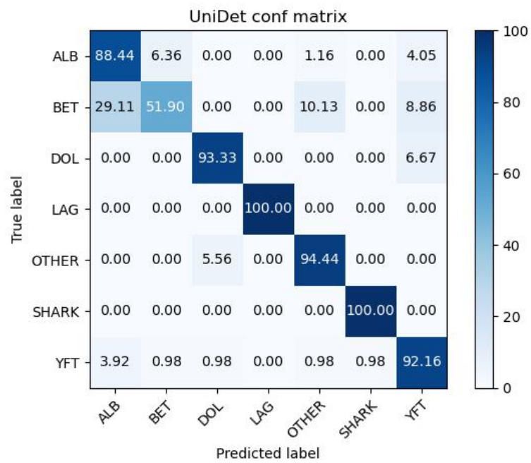
FIGURA 5.12: Matriz de confusión para el testeo del pipeline con UniDet preentrenado
