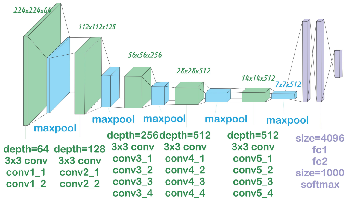
FIGURA 2.5: Versión simplificada de VGG19 [12].
