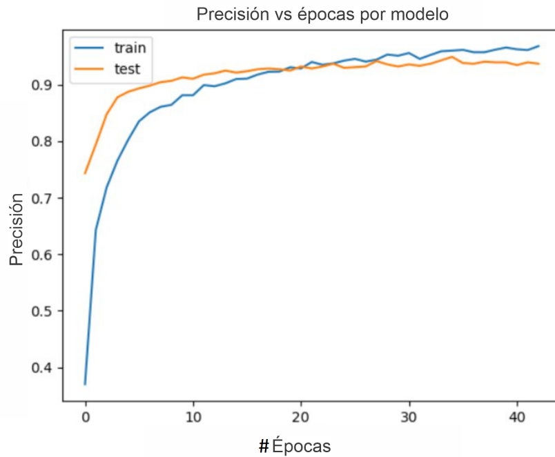
FIGURA 5.6: Gráfica comparativa de la precisión de entrenamiento y validacion
