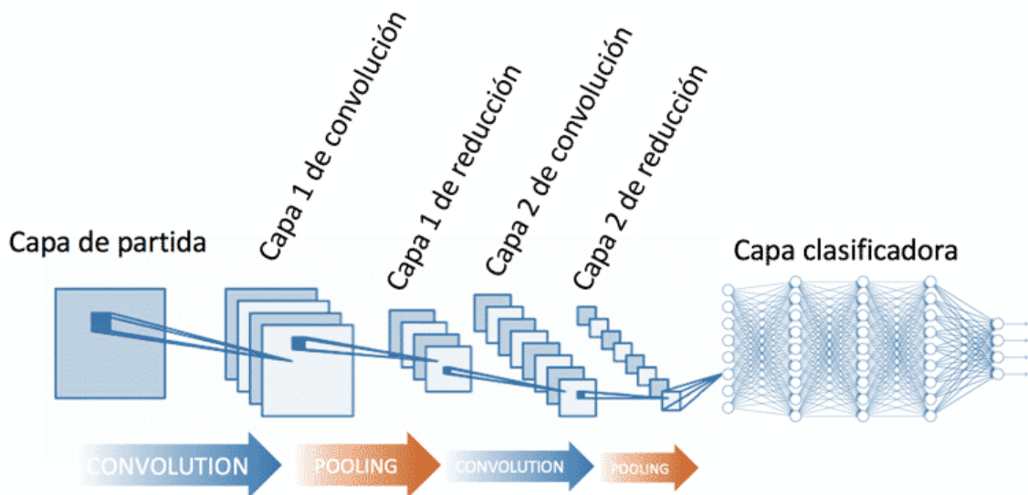
FIGURA 2.4: Arquitectura general de una CNN[10].
