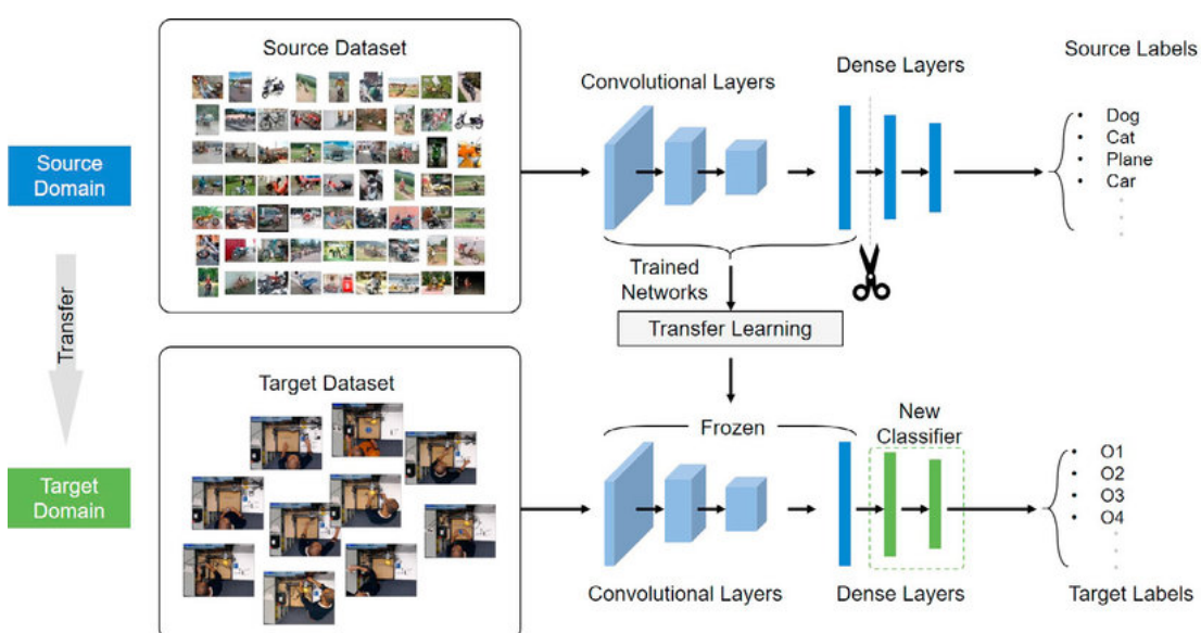
FIGURA 2.13: Comparación entre el aprendizaje común y transfer learning. [22]
