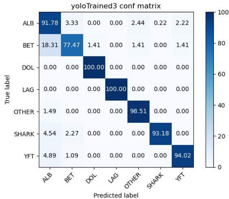
FIGURA 5.13: Matriz de confusión para el testeo del pipeline con Yolov5 entrenado
