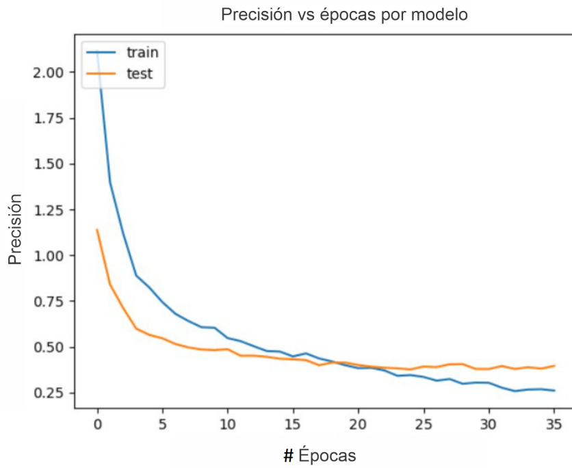
FIGURA 5.8: Gráfica comparativa de la precisión de entrenamiento y validación del experimento #3
