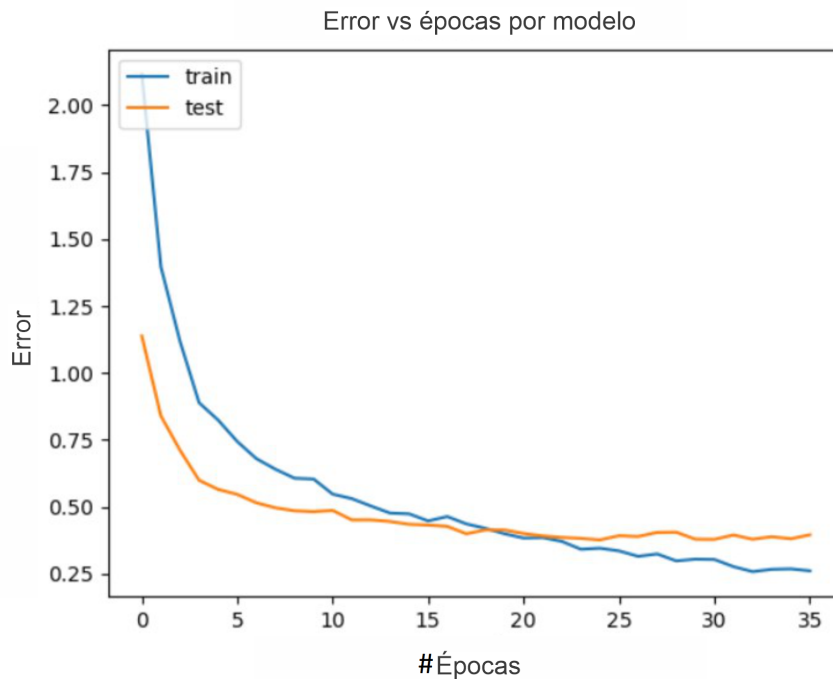
FIGURA 5.7: Gráfica comparativa de la pérdida de entrenamiento y validación del experimento #3
