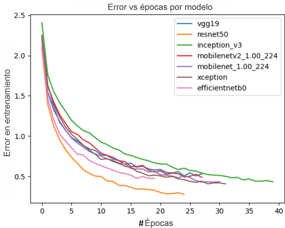
FIGURA 5.2: Gráfica comparativa de la pérdida entre todos los modelos a estudiar
