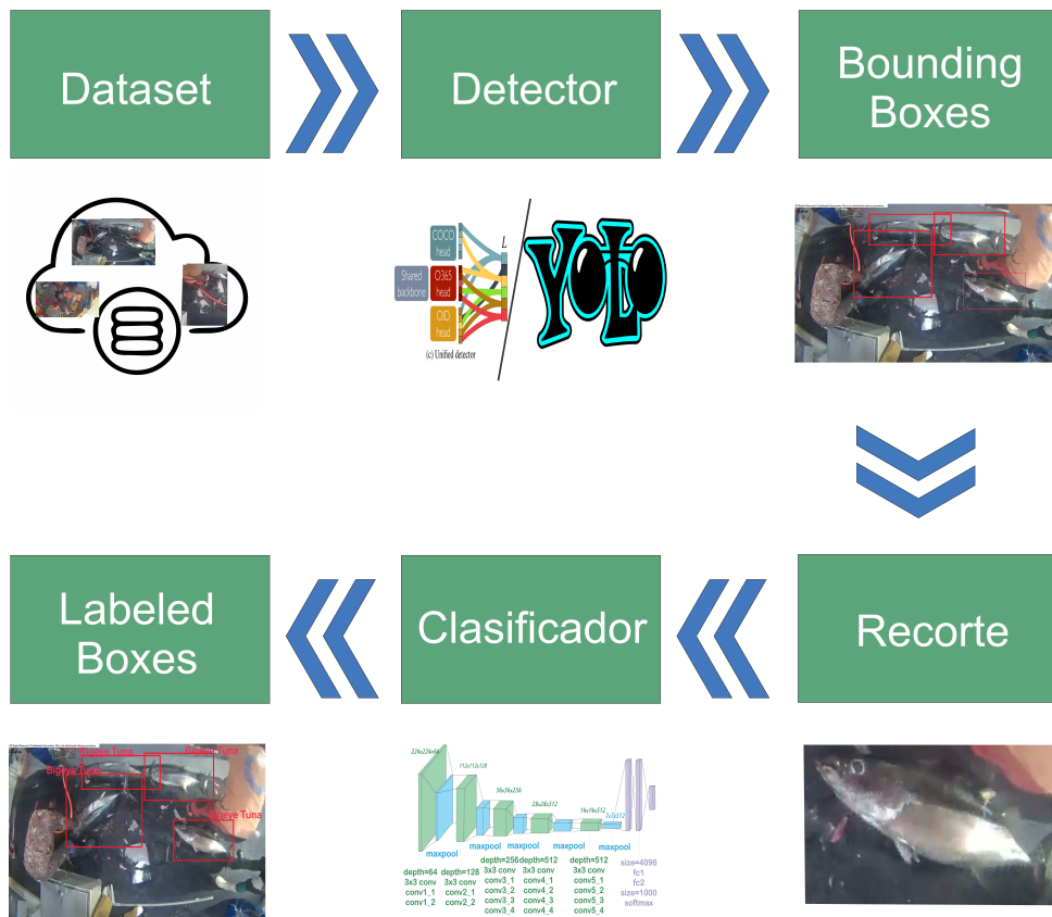
FIGURA 4.1: Pipeline propuesto.
