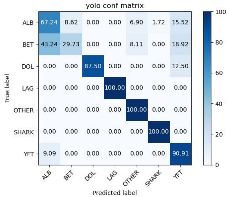
FIGURA 5.9: Matriz de confusión generada por el experimento #3 en porcentajes
