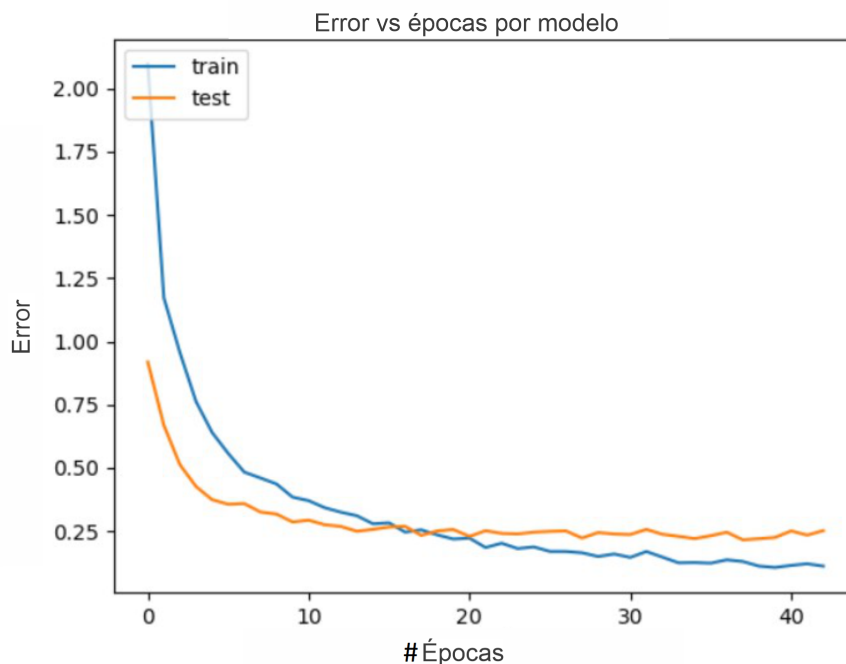
FIGURA 5.5: Gráfica comparativa de la pérdida de entrenamiento y validacion
